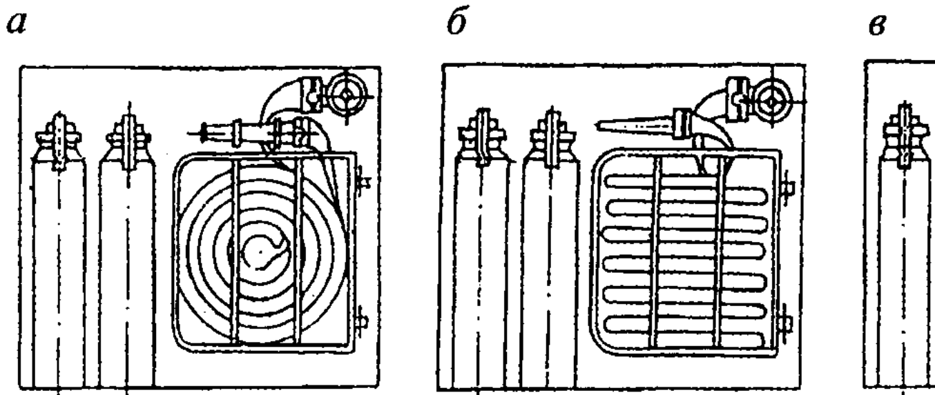
Рисунок 1. Схемы размещения комплектующих изделий
