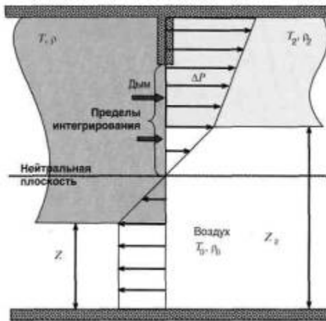
Рис. П6.1 Массопотоки через проем
