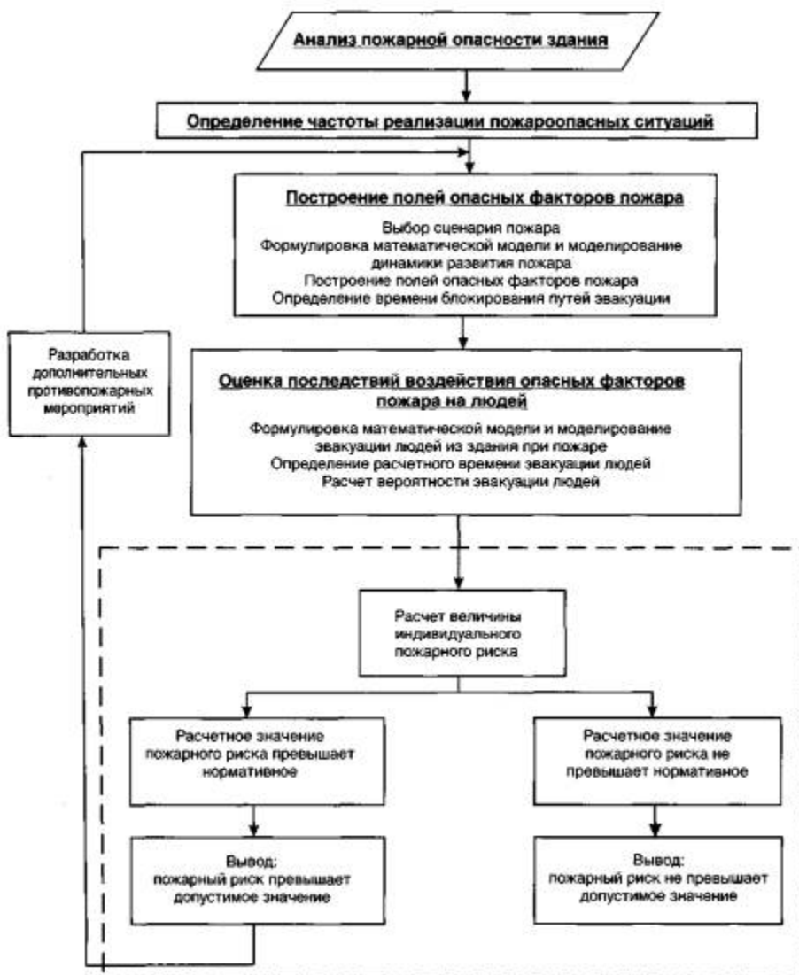
Рис. 1. Порядок проведения расчета индивидуального пожарного риска
